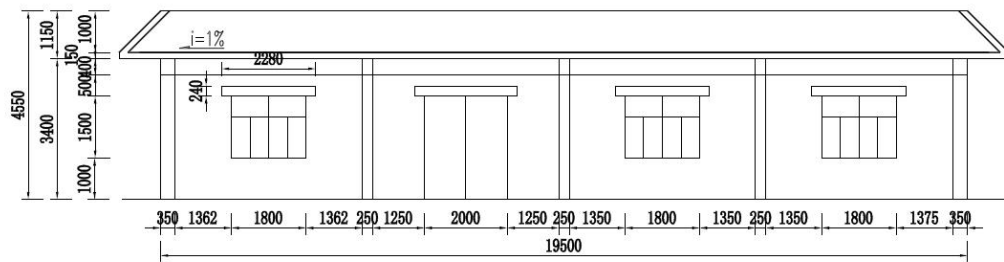
小型泵房II立面图 1:100
