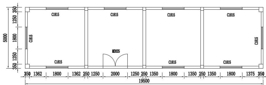
小型泵房II平面图 1:100
