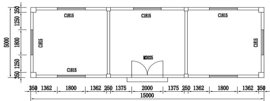
小型泵房 I 平面图 1:100
