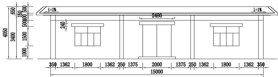
小型泵房 I 立面图 1:100
